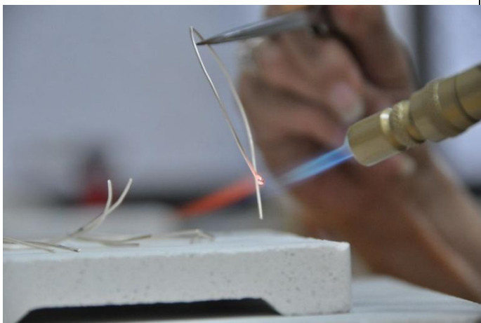
用焊槍燒珠
